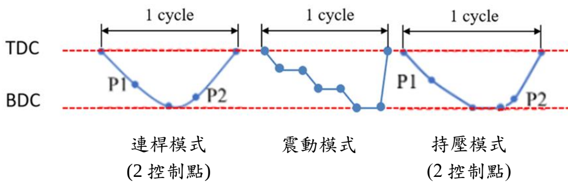
圖 3 基本伺服沖壓運動控制曲線
